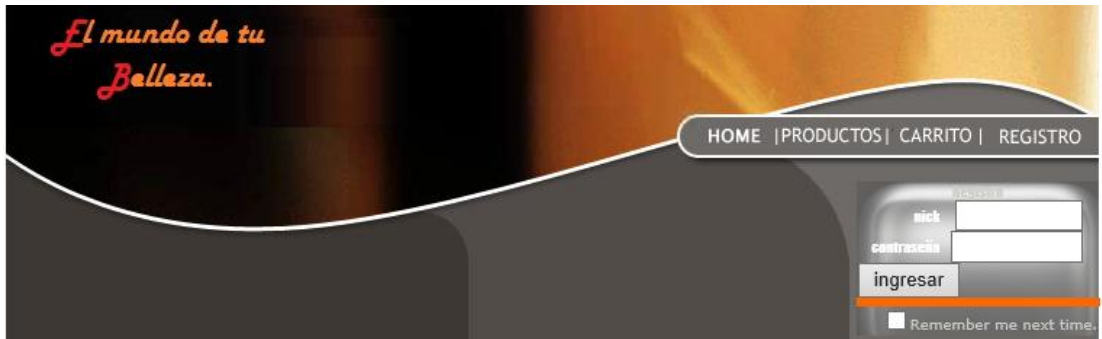
Ilustración 3 - Autenticar
